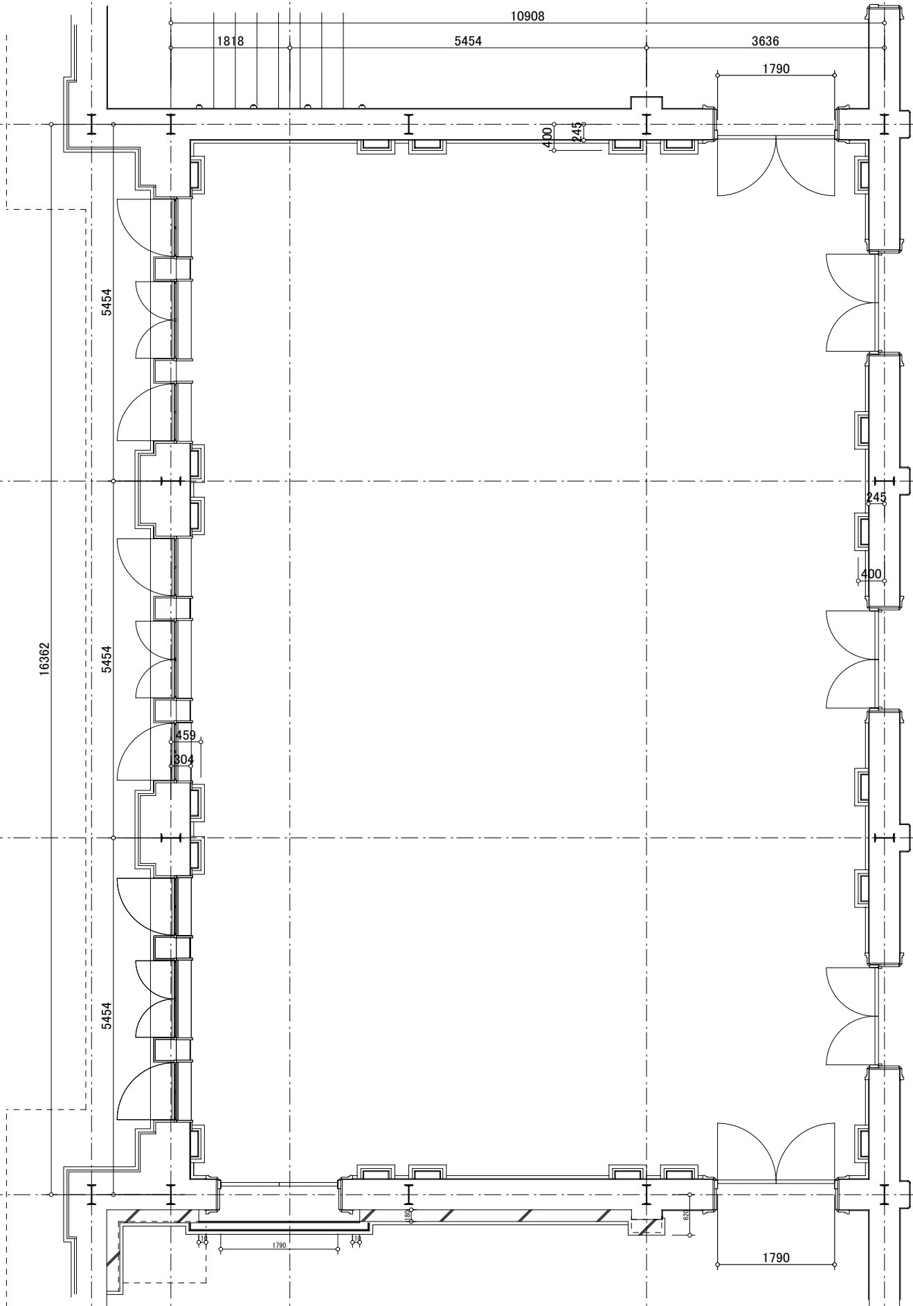
小集会室平面図 1:80
